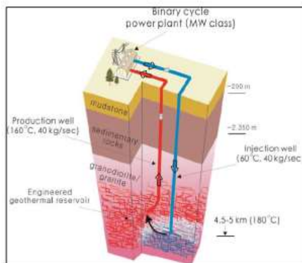
第 8.2 図 韓国の EGS パイロットプラントプロジェクトの概念図
