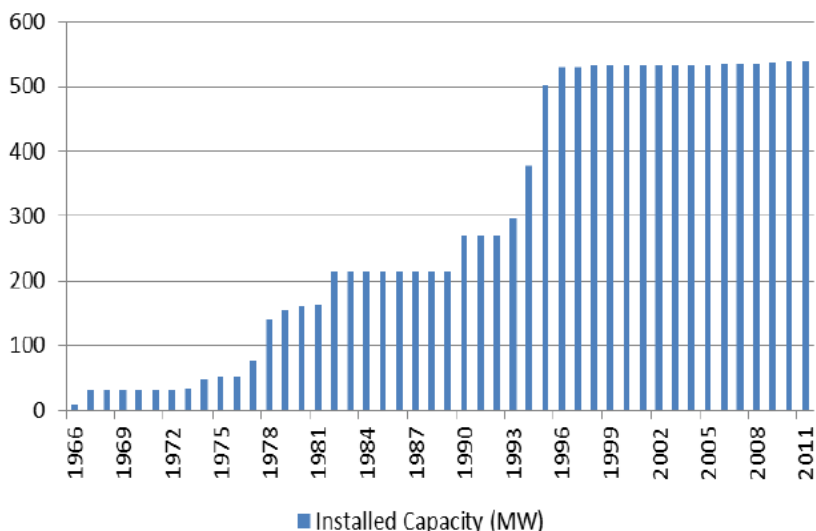
第 7.1 図 日本における地熱発電プラントの全設備容量
