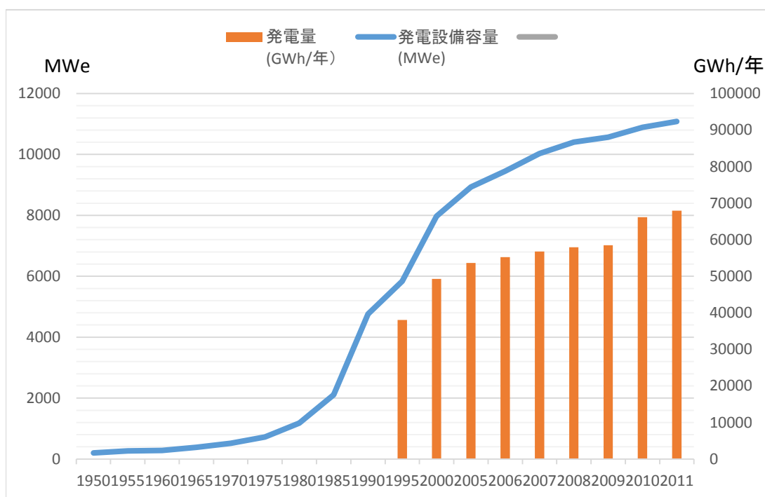
第 1-2 図 世界における 1950 年から 2011 年までの地熱設備容量と 1995 年から 2011 年までの発電量
