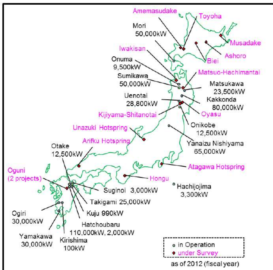
第 7.3 図 2012 年現在の日本の地熱プロジェクト
