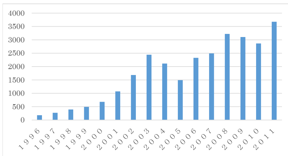
第 11.1 図 1996 年から 2011 年までの年間水/水ヒートポンプ設置台数。 空気/水ヒートポンプの設置台数も同様な傾向を示している。
