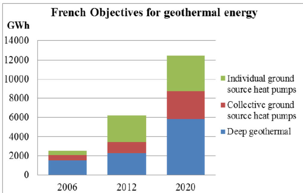
第 3.2 図 フランスにおける地熱暖房の将来の動向
