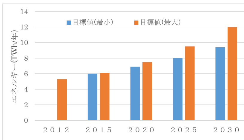
第 6.6 図 イタリアにおける地熱発電の将来予測
