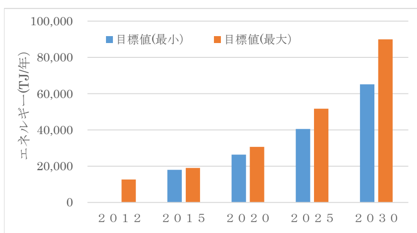
第 6.7 図 イタリアにおける地熱直接利用の将来予測
