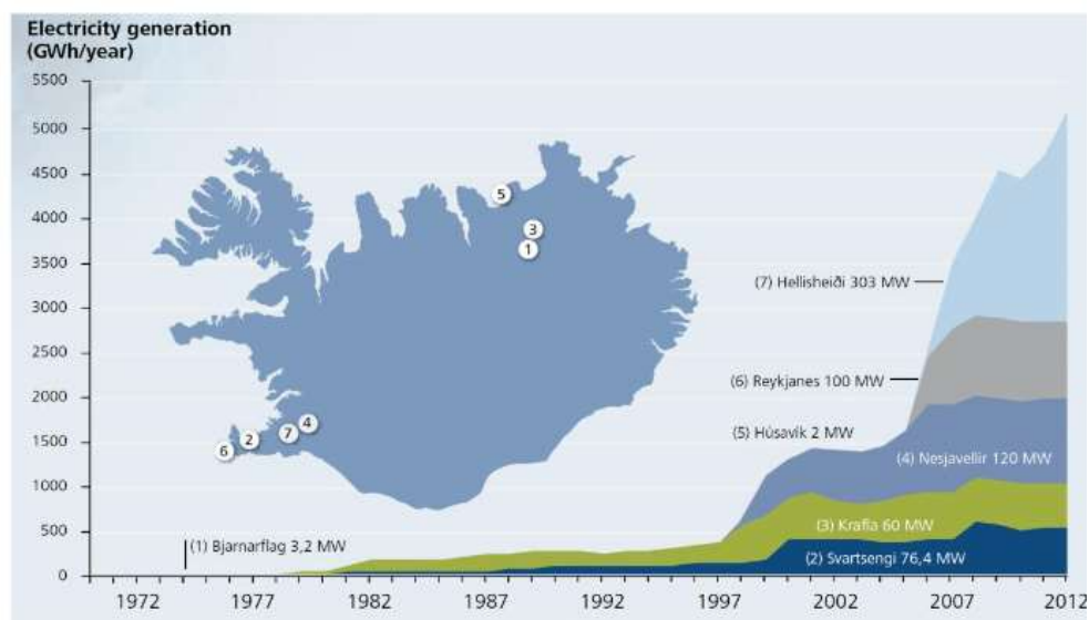
第 5.4 図 1969 年から 2012 年のアイスランドにおける地熱発電の推移
