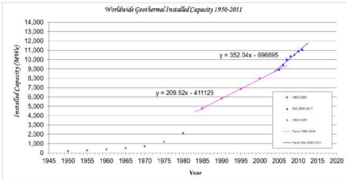
第 1-3 図 世界における 1945 年から 2011 年までの地熱発電設備容量の推移
