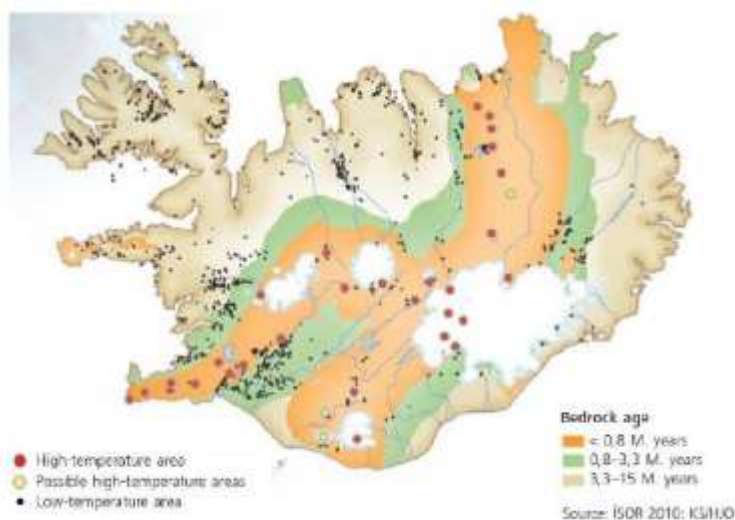
第 5.2 図 アイスランド火山地帯の高温地熱フィールドと火山の山腹の低温泉クラスター位置。アイスランドは、ホットスポットと大西洋中央海嶺上に位置しており、地質的に非常に活発である。
