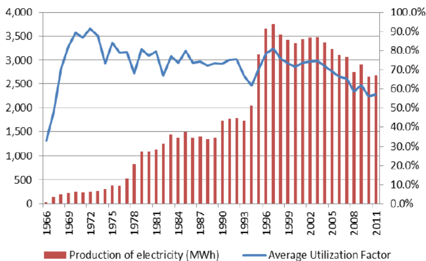
第 7.2 図 日本における地熱発電の全発電量と平均利用率
