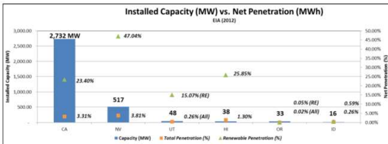
第 15.3 図 それぞれの州における地熱の市場浸透
