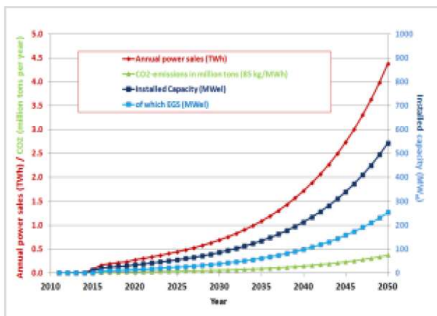
第 13.2 図 スイスの地熱発電成長のシナリオ。このシナリオは、地熱エネルギーからの電力を推進するという政策手段をもとに作成された。
