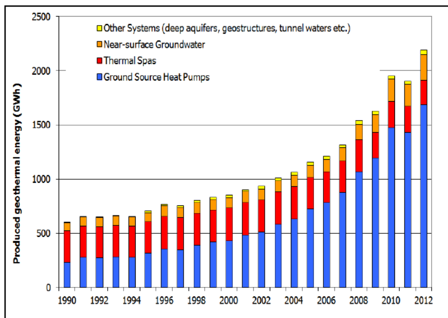
第 13.1 図 スイスにおける地熱エネルギー利用の現状
