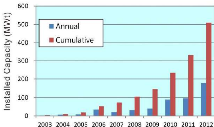
第 8.1 図 増加傾向を示す GHP 設置台数
