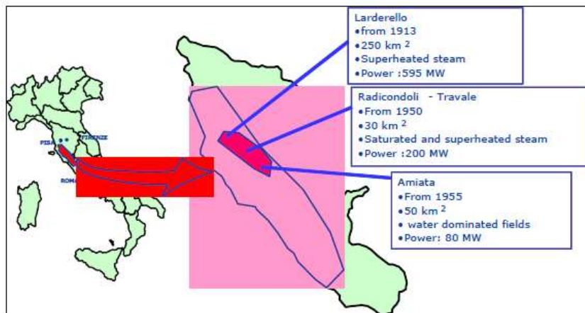
第 6.2 図 イタリアの地熱地帯
